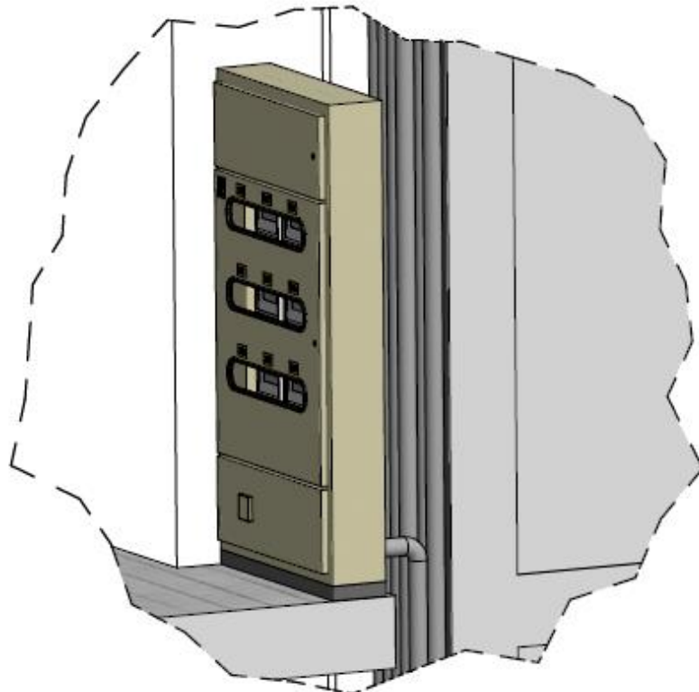
Figura 2B. Detalle B de la Figura 2, Tablero de Medida de Piso.
