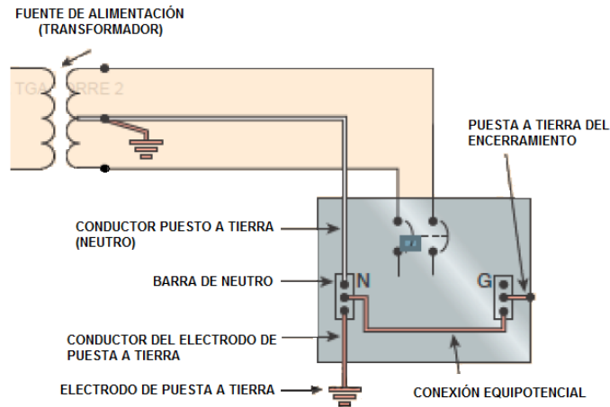
Figura 7. Conexión equipotencial en tablero principal.
