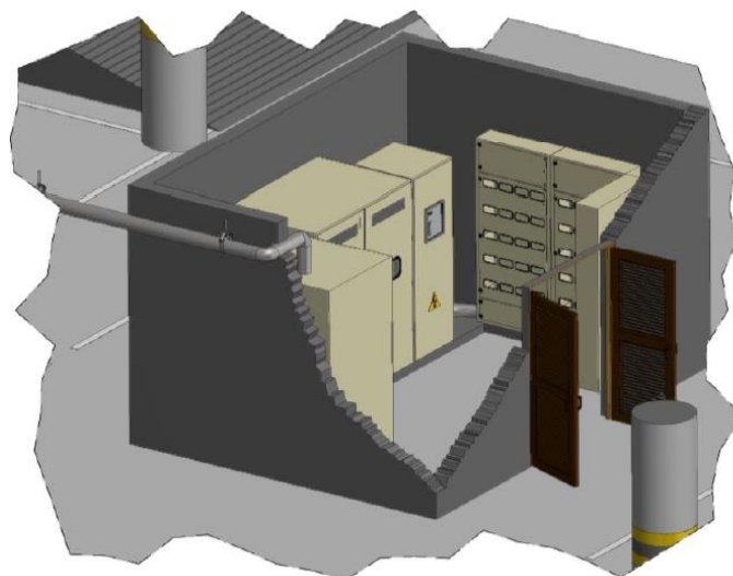
Figura 1. Tablero de medida concentrada en cuarto técnico.
