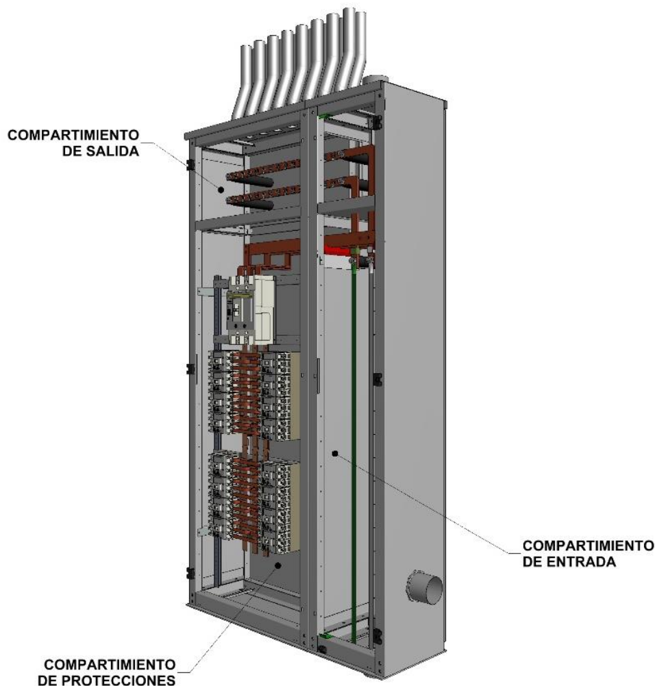
Figura 14. Compartimientos Tablero General de Alimentadores - TGA
