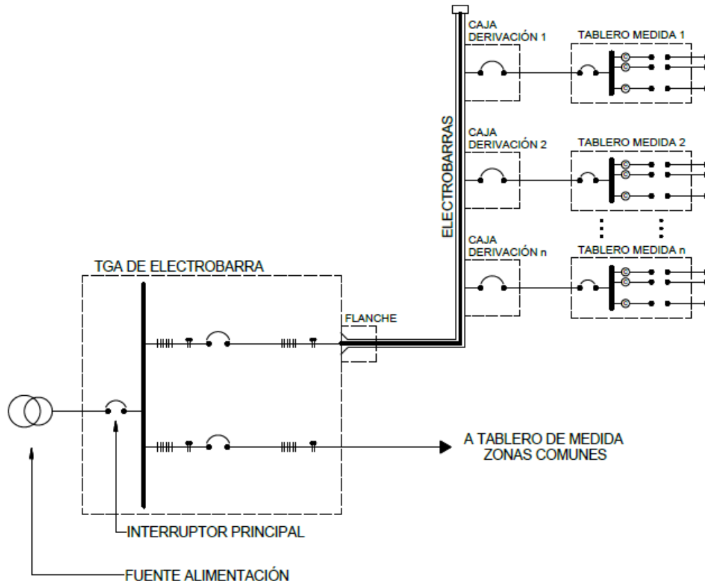
Figura 3. Diagrama unifilar ilustrativo para medida descentralizada por medio de electrobarra.
