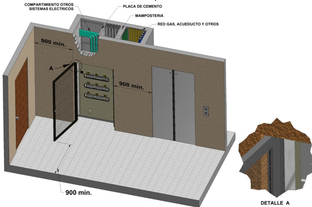
Figura 10. Características del buitrón y separación mínima de puertas y tableros a diferentes accesos, muros o salidas.
