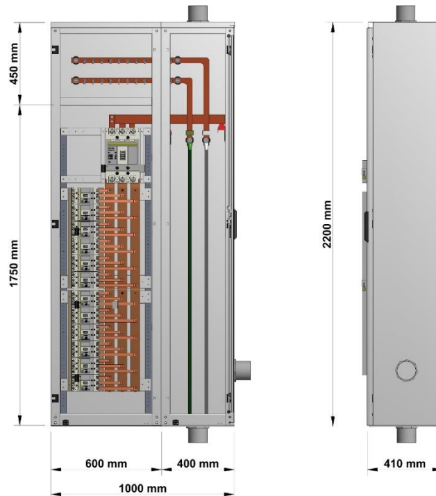
Figura 16. Dimensiones TGA con una columna de interruptores.
