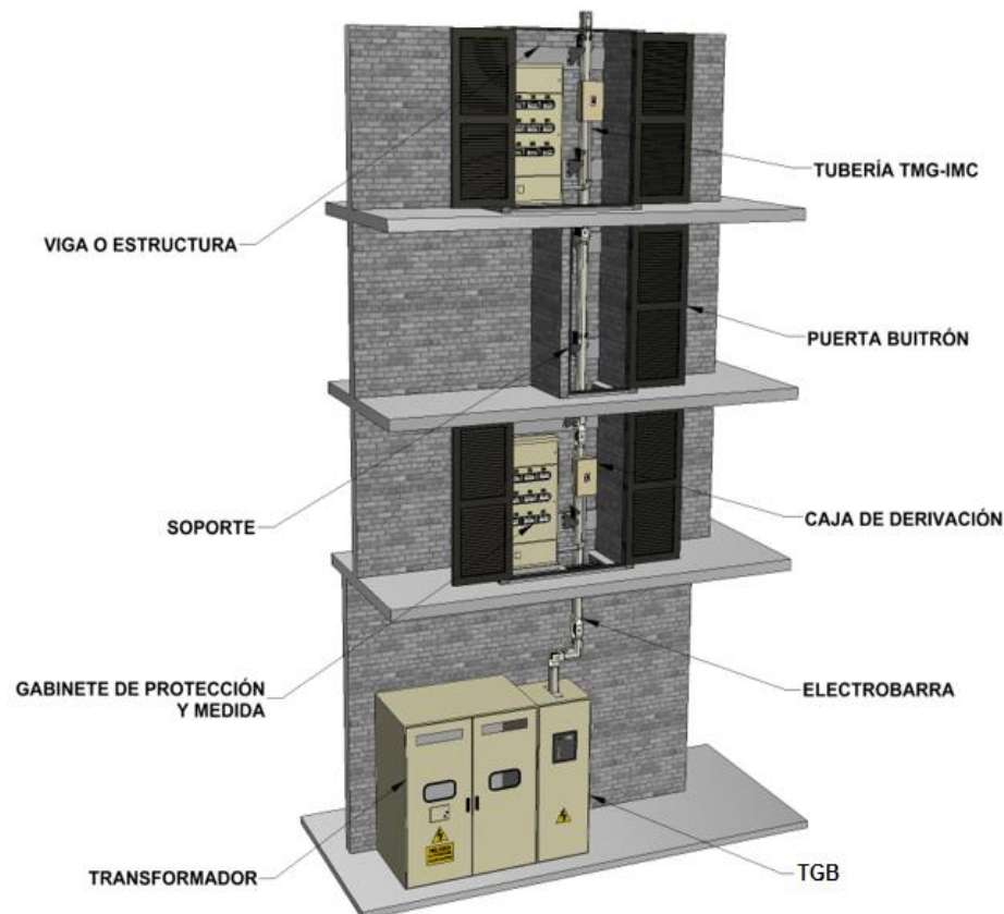
Figura 4. Esquema ilustrativo para medida descentralizada con bus de barras desde la subestación a los tableros de medida.
