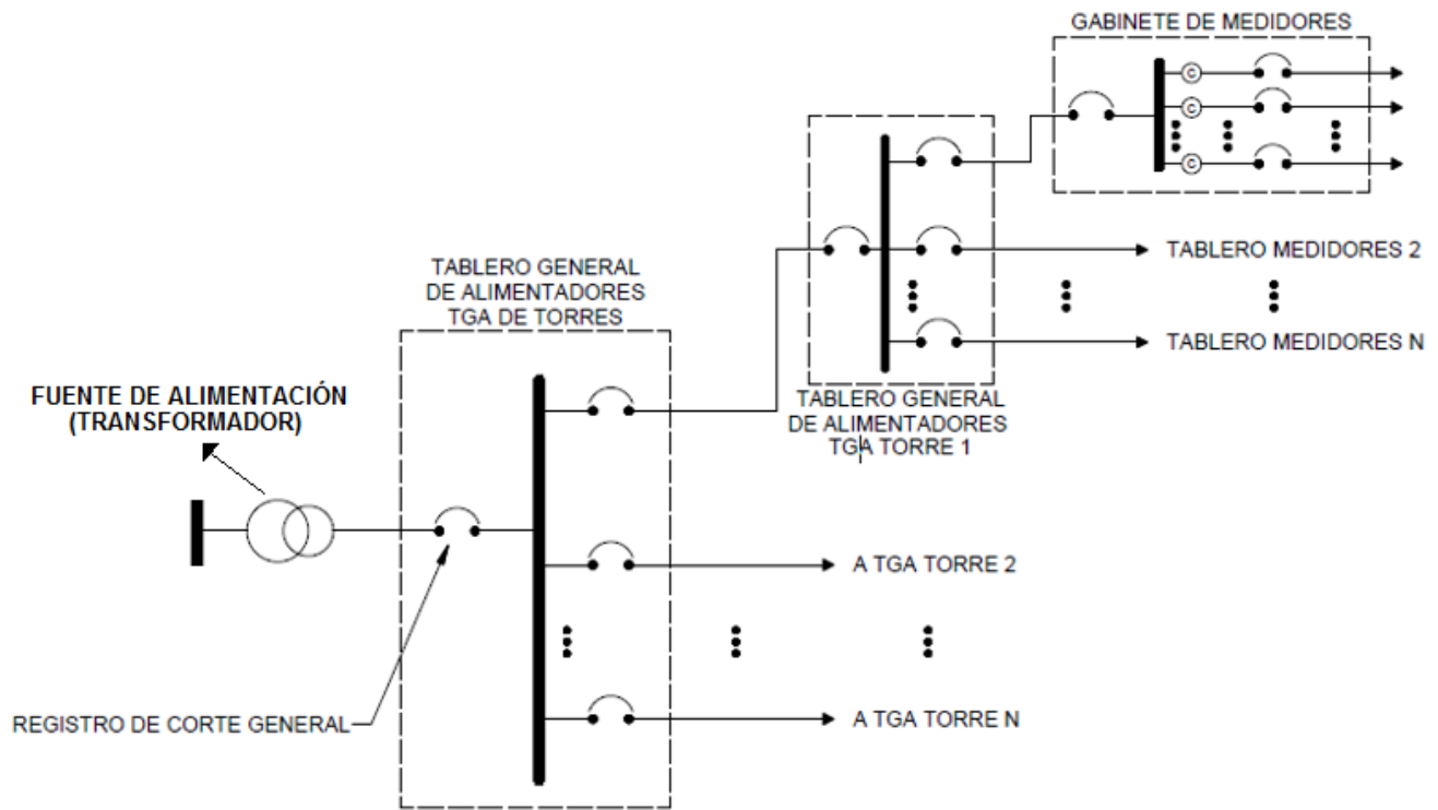
Figura 6. Diagrama unifilar ilustrativo para medida descentralizada por medio de cables convencionales para varios Tableros Generales de Alimentadores.
