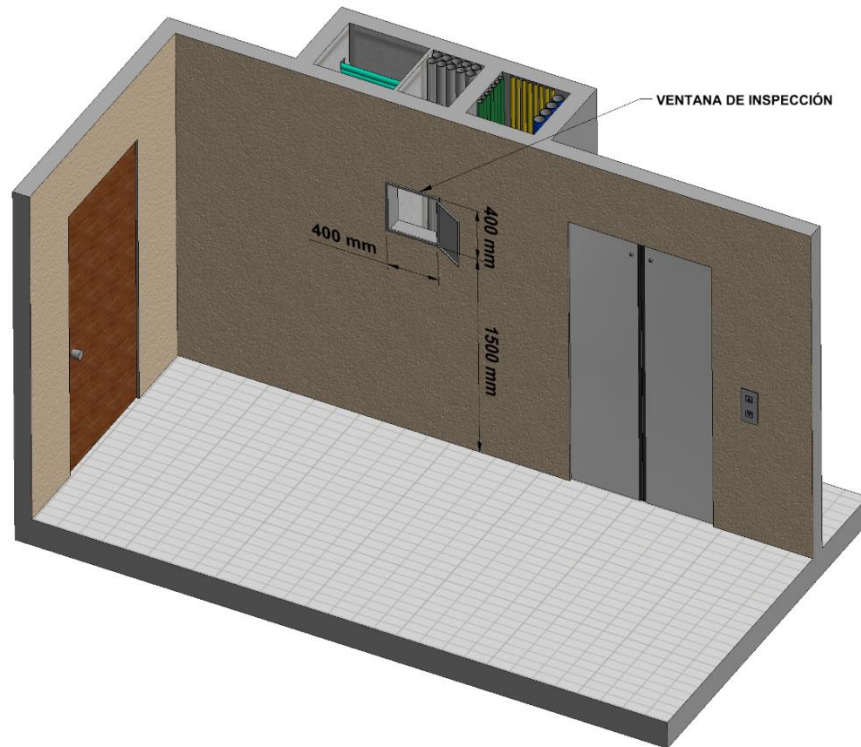
Figura 11. Ventana de inspección
