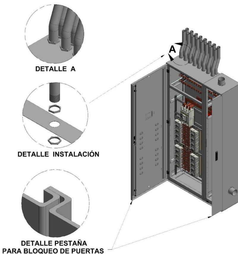
Figura 17. Instalación de los ductos que ingresan al tablero y detalle para bloqueo de puerta del compartimiento de entrada en los Tableros Generales de Alimentadores – TGA.
