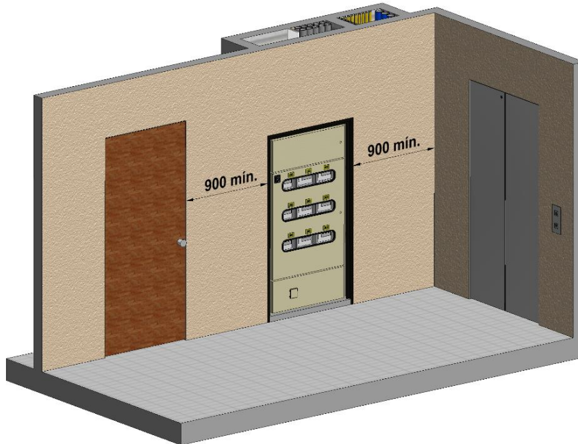
Figura 10. Características del buitrón y separación mínima de puertas y tableros a diferentes accesos, muros o salidas.
