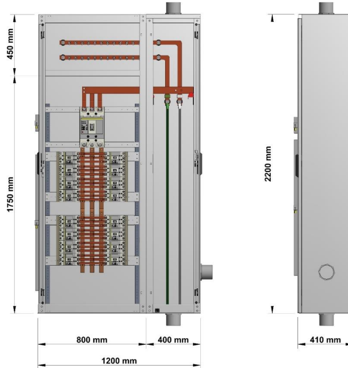
Figura 16. Dimensiones TGA con una columna de interruptores.
