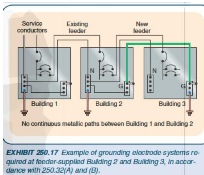
Figura 8. Conexión equipotencial en tableros principales para dos o más edificaciones alimentados desde una acometida común.
