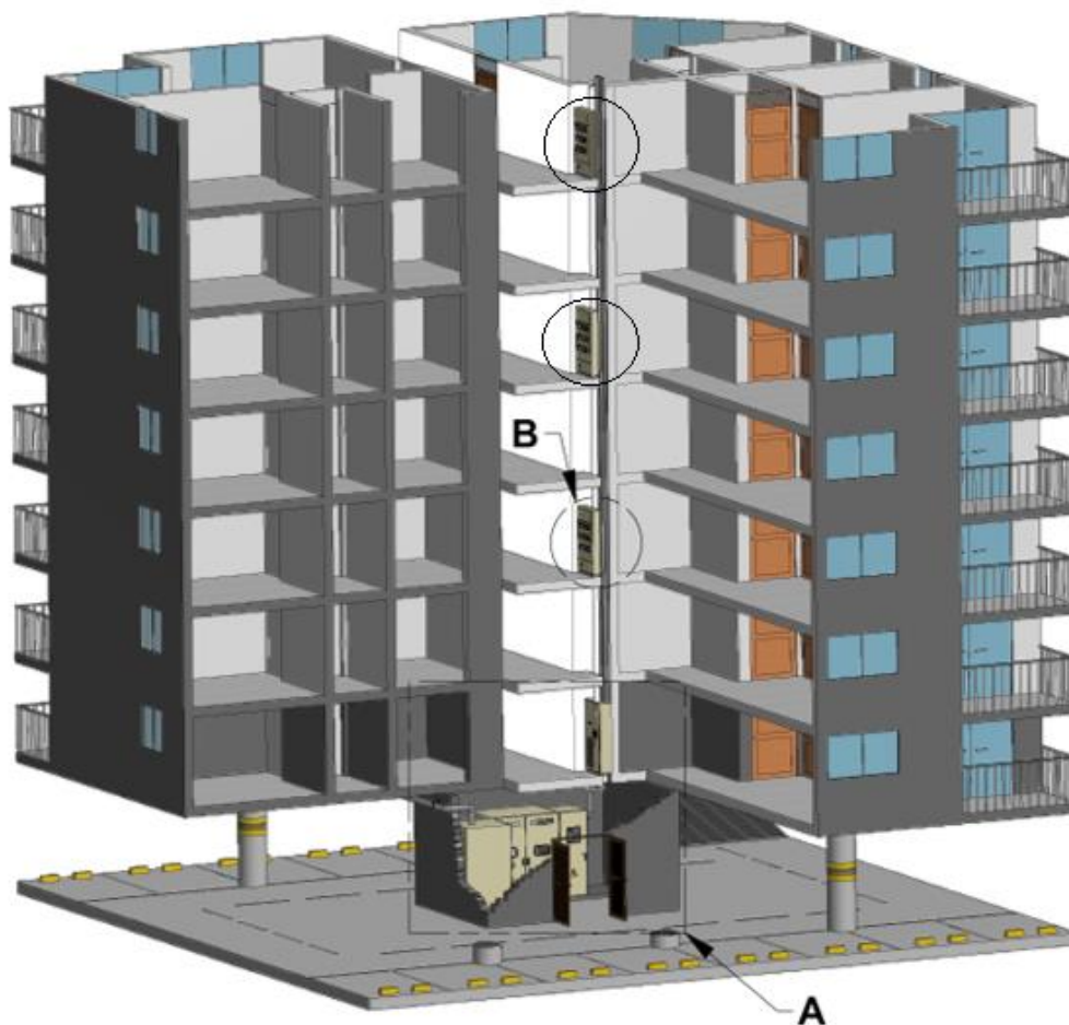
Figura 2. Sistema de medida distribuida con tableros ubicados en diferentes niveles de la edificación
