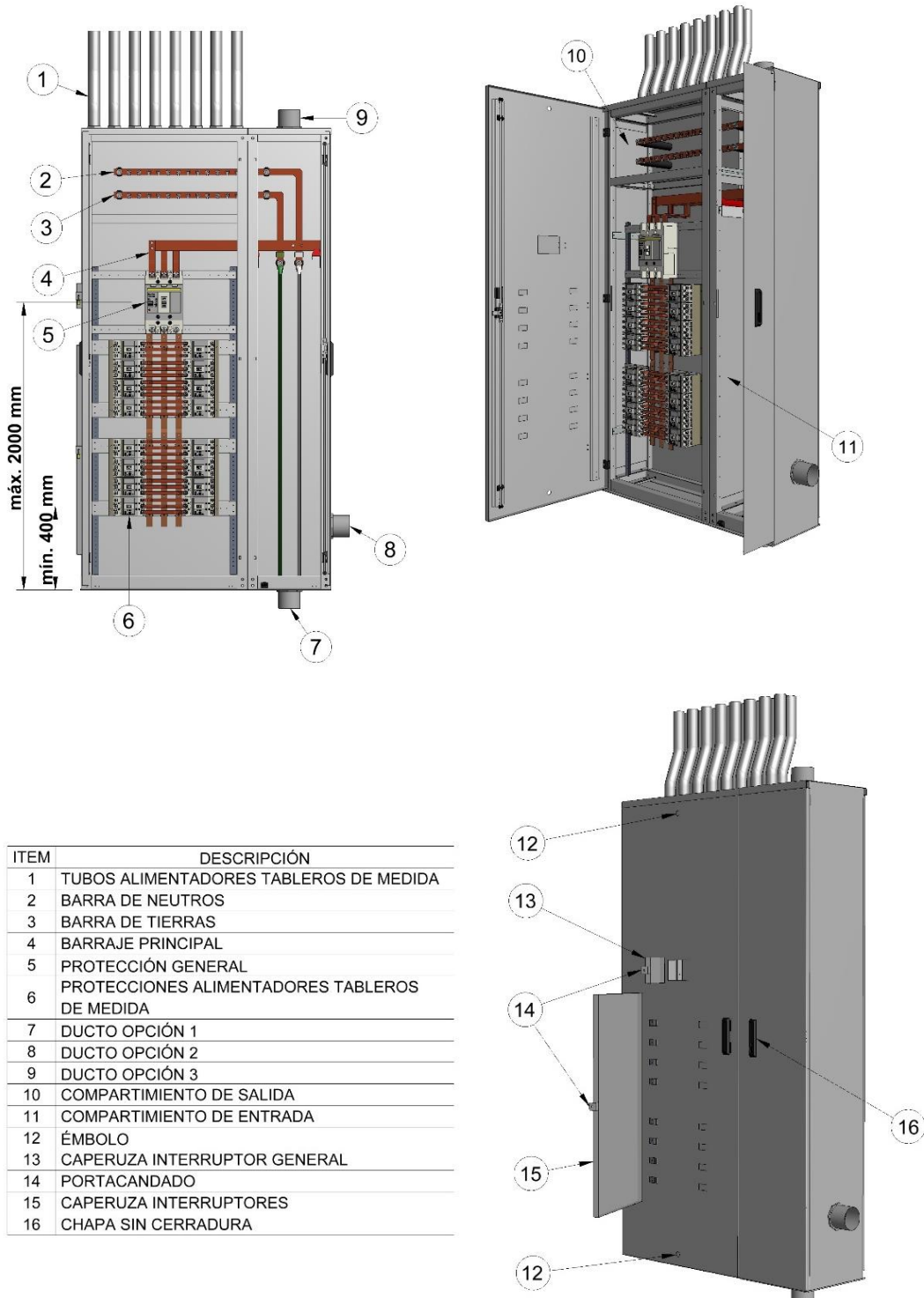
Figura 18. Identificación de componentes en los Tableros Generales de Alimentadores – TGA
